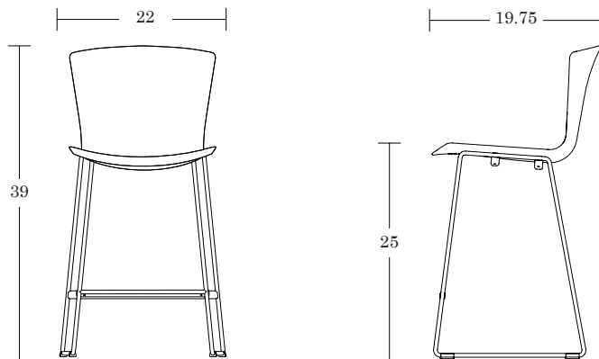
Sled Base Counter Chair / SLCS
